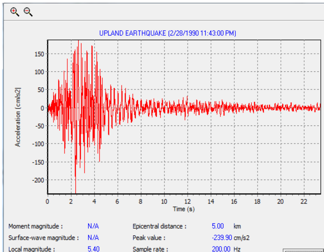
Fig. 4: Accelerogram.
